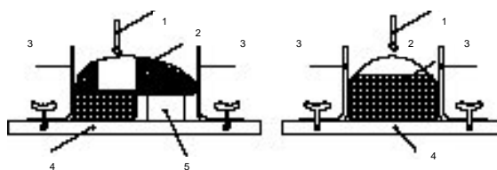
1 Tige et sphère 2 Masque 3 Eléments de blocage à coulisse 4 Base fixe de l'appareil d'essai 5 Support pour maintenir le masque en position
